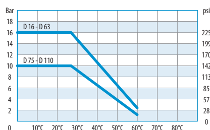
VARIACIÓN DE LA PRESIÓN EN FUNCIÓN DE LA TEMPERATURA PARA AGUA Y LÍQUIDOS NO AGRESIVOS
