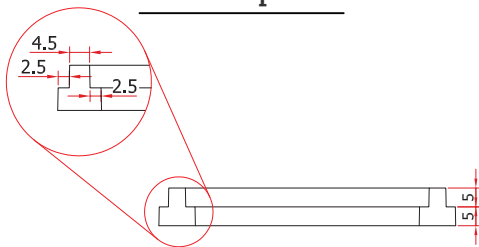
Vista Frontal en corte
